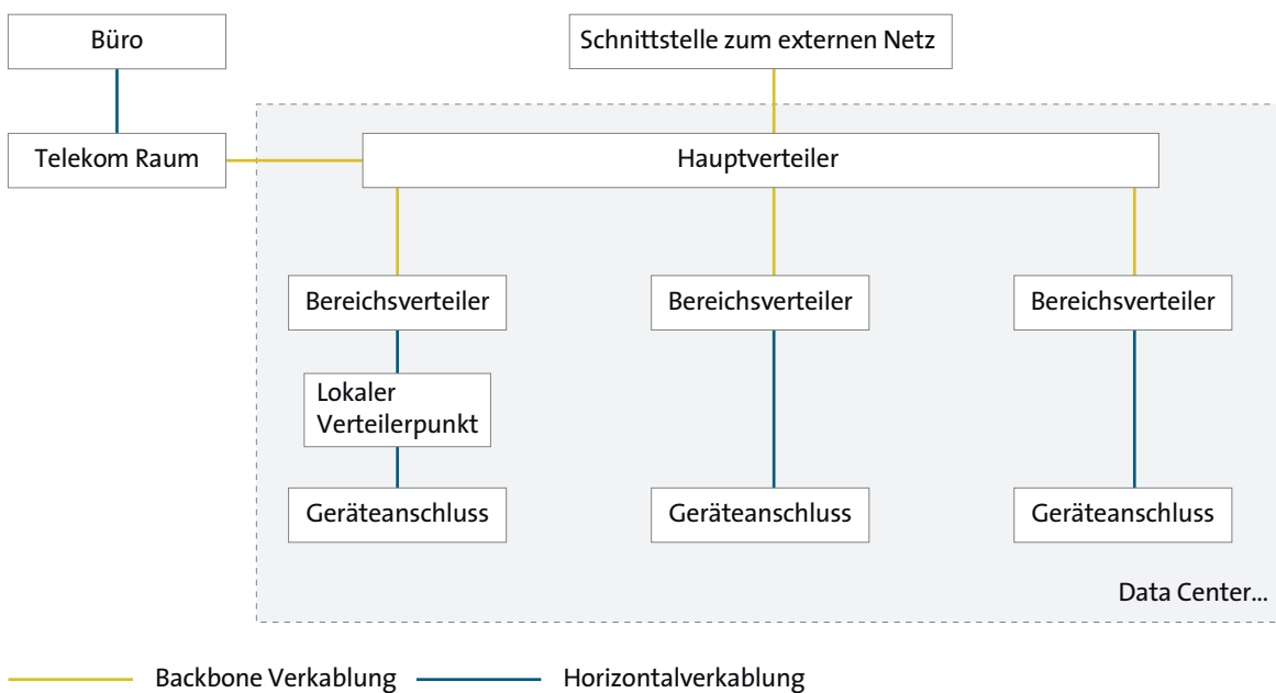
Abbildung 10: Schematische EN 50173-5 / TIA 942 Verkabelungsstruktur
