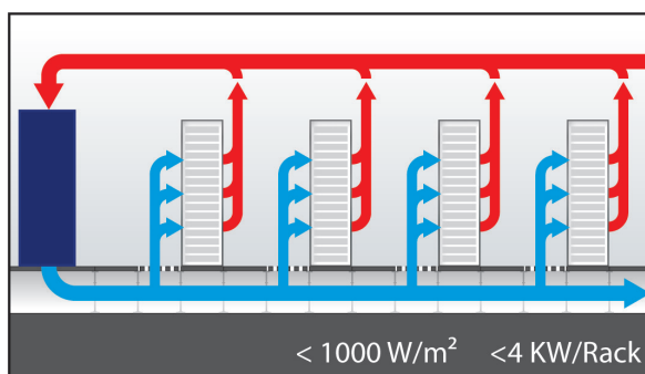
Klimatisierung über den Doppelboden ohne Ordnung der Racks aus lüftungstechnischer Sicht
