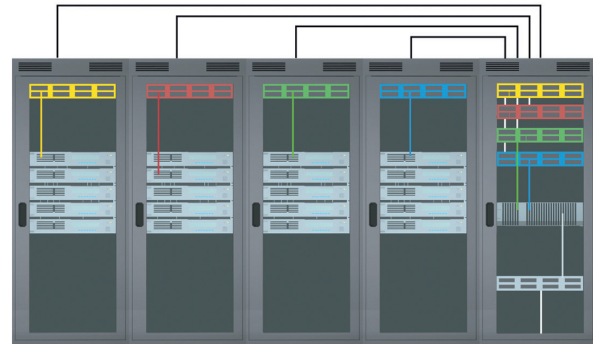
Abbildung 11: Darstellung: Horizontalverkabelung (Cu und LWL) mit Bereichsverteiler (BV) und Server-/Storageschränken mit Geräteanschluss (GA)
