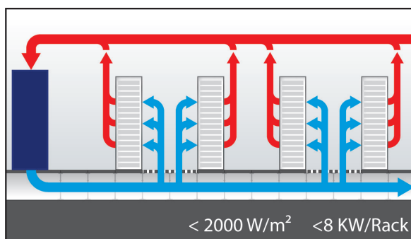
Klimatisierung über den Doppelboden und Einhausung der Kaltgänge
