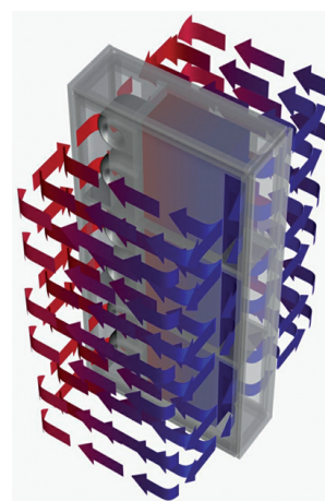
Abbildung 7: Prinzipielle Darstellung wassergekühltes Serverrack
