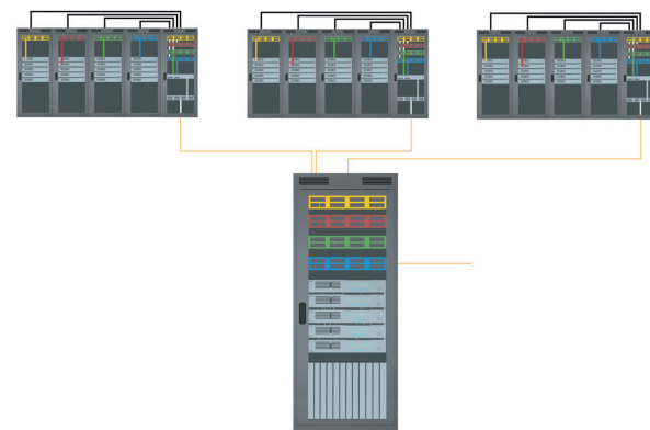
Abbildung 12: Darstellung: Backboneverkabelung (LWL) mit Hauptverteiler (HV) und Anschluss an die Horizontalverkabelung (Cu und LWL) mit Bereichsverteiler (BV) und Server-/Storageschränken mit Geräteanschluss (GA)
