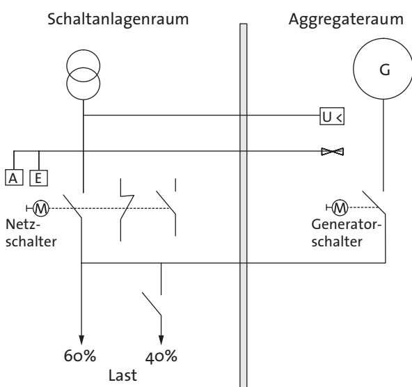
Abbildung 5: Netzüberwachung / Netzschnittschaltung
