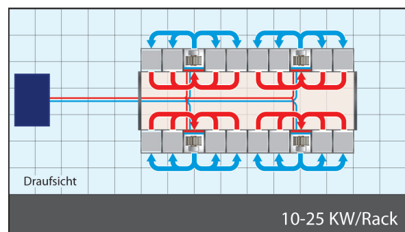
Klimatisierung wassergekühlt Einhausung der Warmgänge
