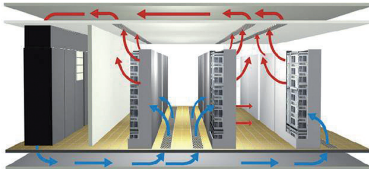
Abbildung 6.: Prinzipielle Darstellung einer Kaltgang-Warmgang Lösung
